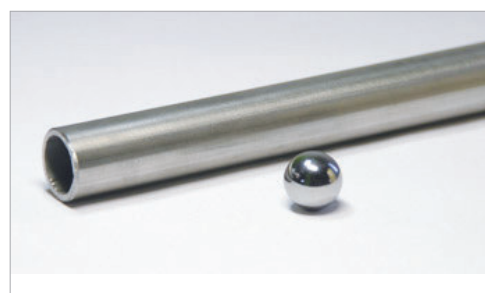
Prüfkegeldruchmesser \varnothing 5/8 Zoll. Länge des Fallrohres 1200 mm.
